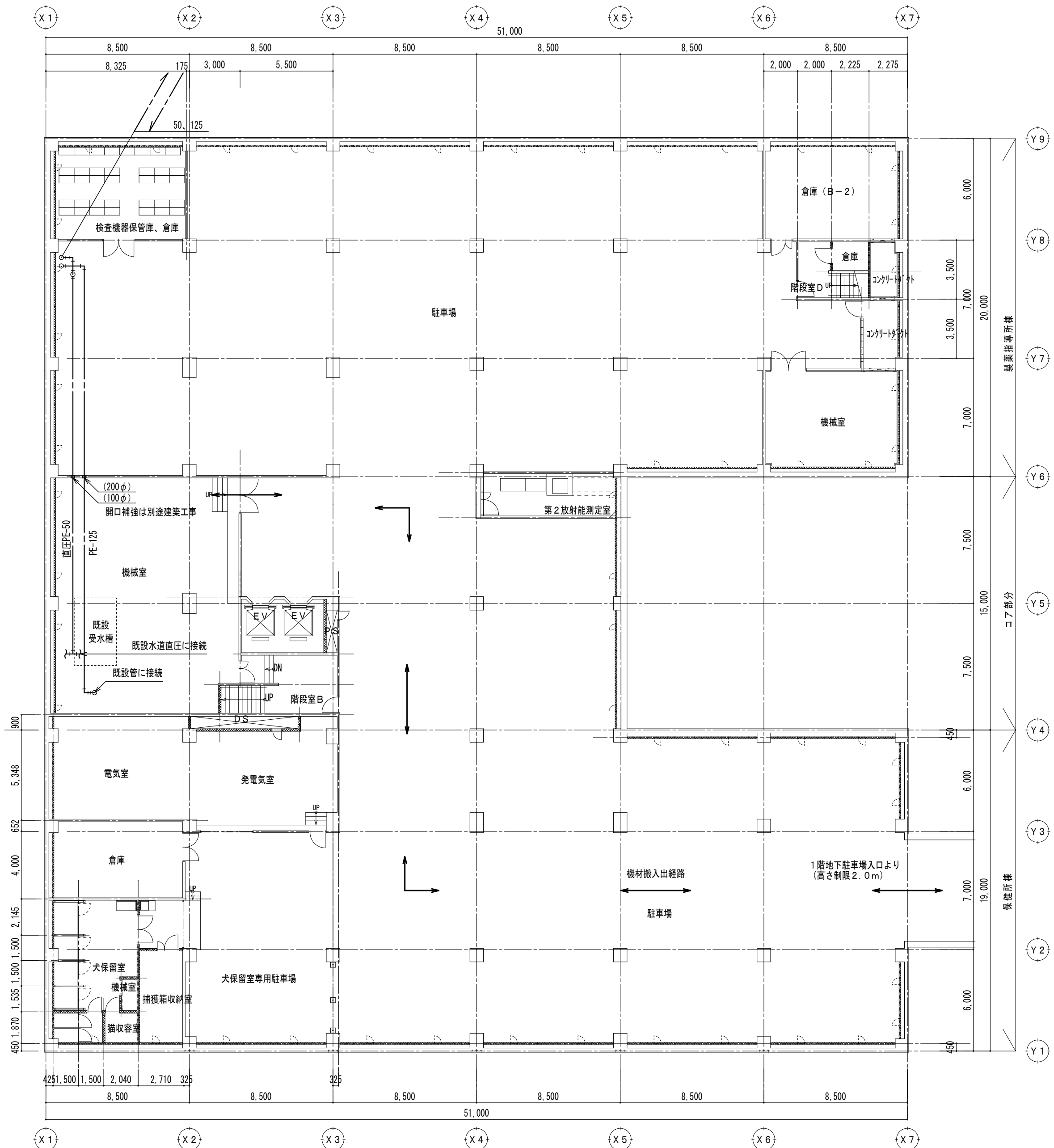
地下1階平面図 S=1/200
